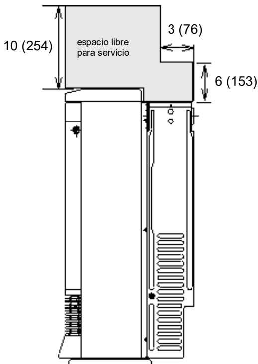
Figura 7. Espacios libres recomendados para tareas de servicio
