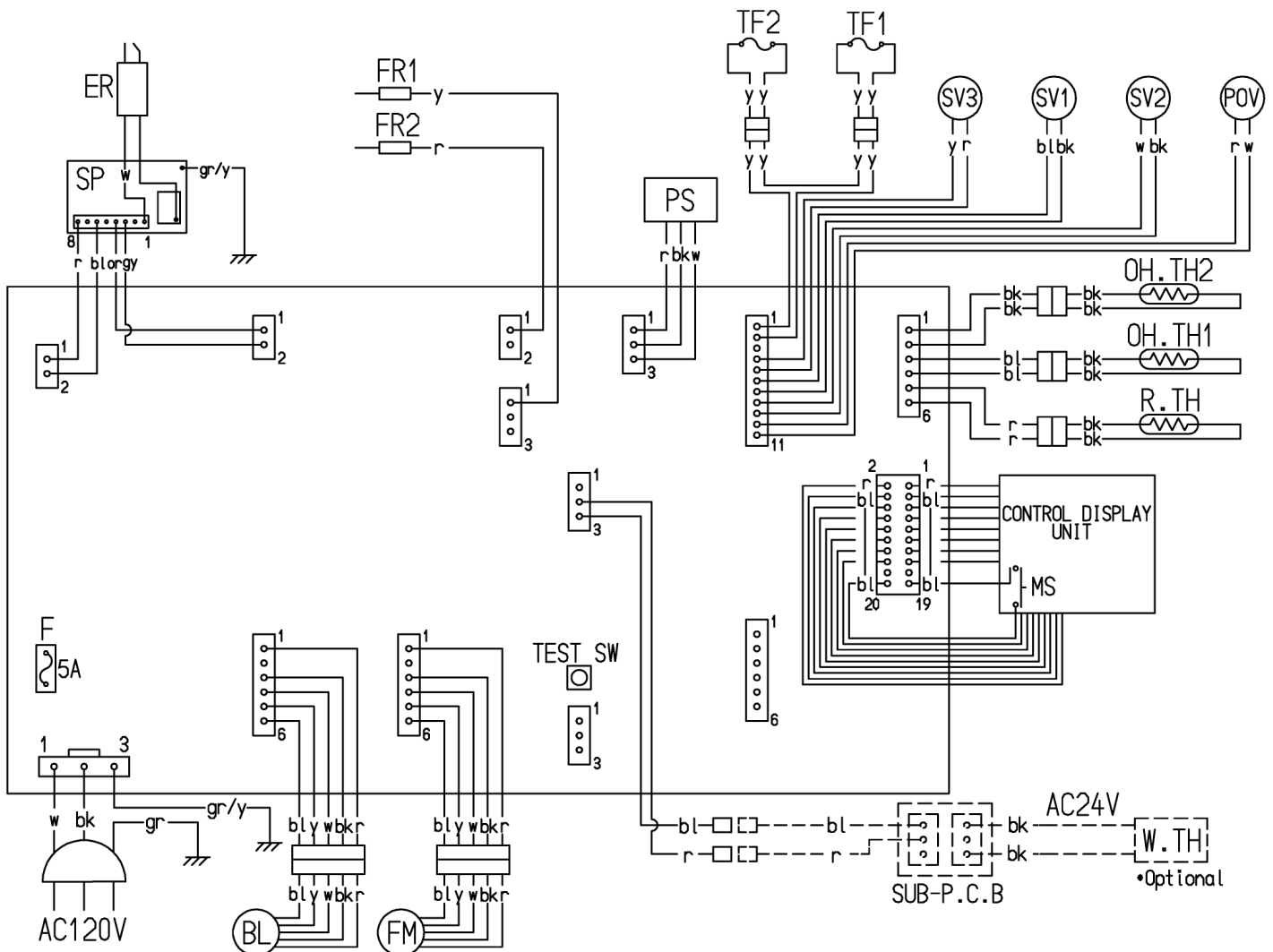
Figura 64. Diagrama de conexionado
